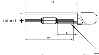
vor dem Kürzen längerer Pin longer pin before shortening
